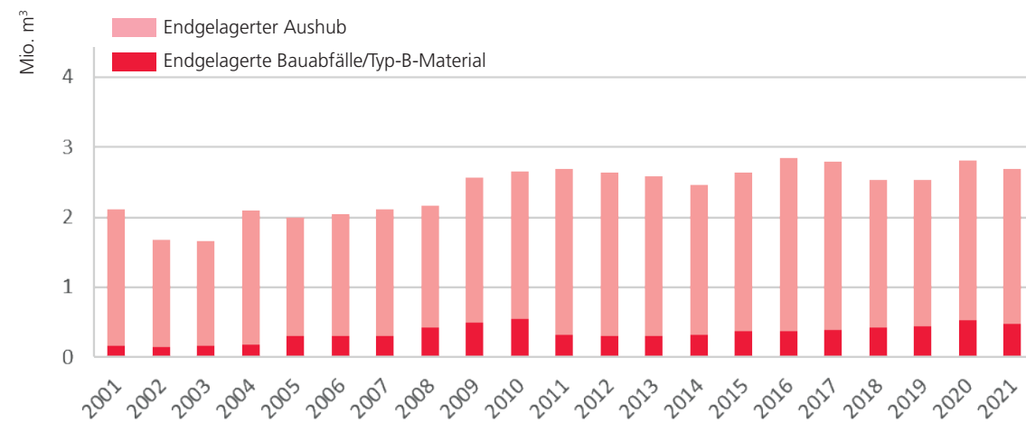
Zur Ablagerung angenommene Mengen an sauberem Aushub und Bauabfällen/Typ B-Material der KSE-Mitglieder [Mio. m³ lose]
