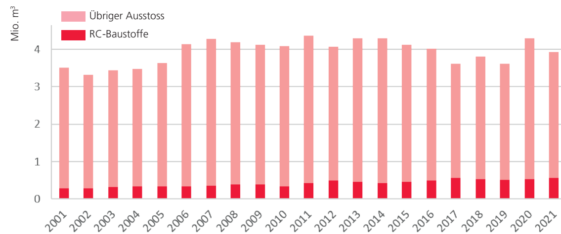
Ausstoss an Gesteinkörnungen (Kies, Sand, Fels, RC-Baustoffe) der KSE-Mitglieder [Mio. m³ lose]
